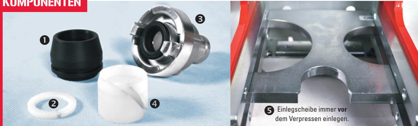
1 Schwarzer Außenring 2 Arretierring 3 Knaggeteil mit Stutzen 4 weißer Innenring (D 25 1,6-2,0 mm Schlauchwandstärke, Bsp. GH TITAN X-TREME) 5 Einlegscheibe mit zusätzlicher Aussparung für D 25.
